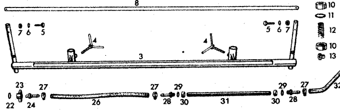
Teile SF 300
